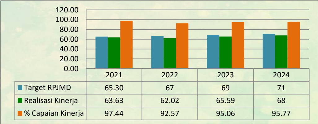
Grafik 3.5 Perbandingan Target RPJMD dengan Realisasi Indikator Kinerja Persentase Tingkat Kondisi Jaringan Jalan Kabupaten Baik dan Sedang Tahun 2021-2024
